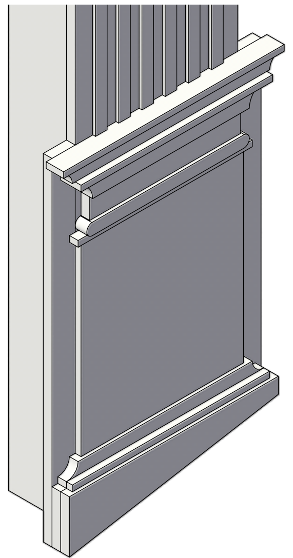
F-5 pilaster: iso Scale: 2" = 1'-0"
