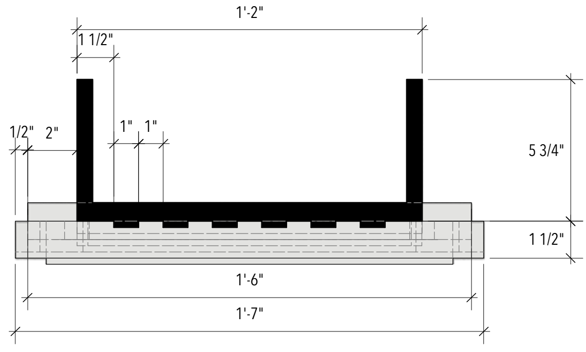
F-2 pilaster: section BB' Scale: 3" = 1'-0"
