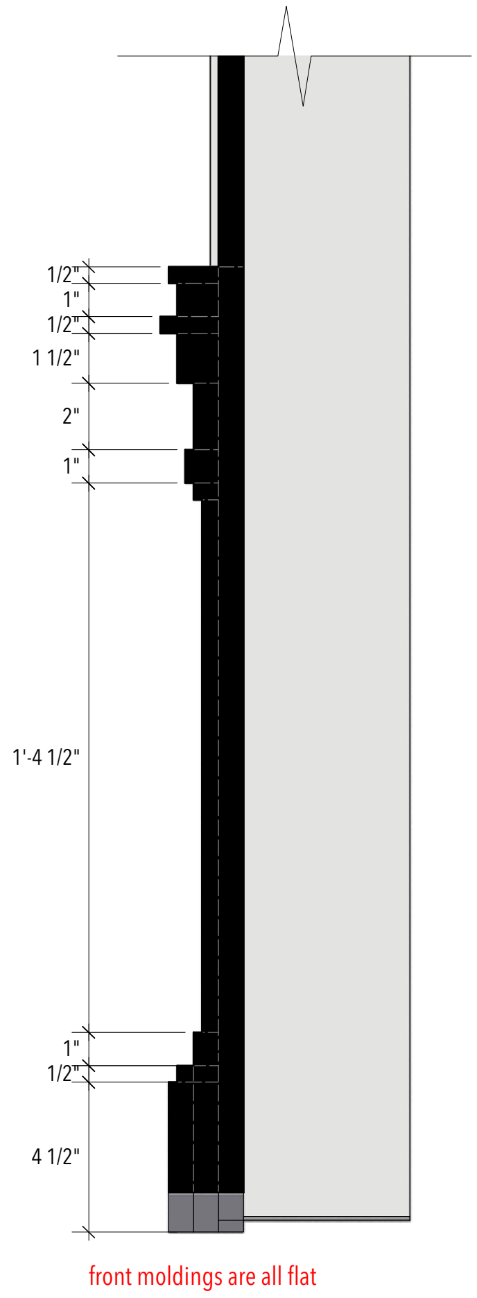
F-3 pilaster: section CC' Scale: 3" = 1'-0"
