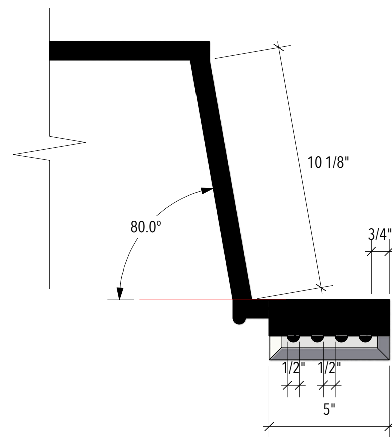
E-7 fireplace section FF' Scale: 3" = 1'-0"
