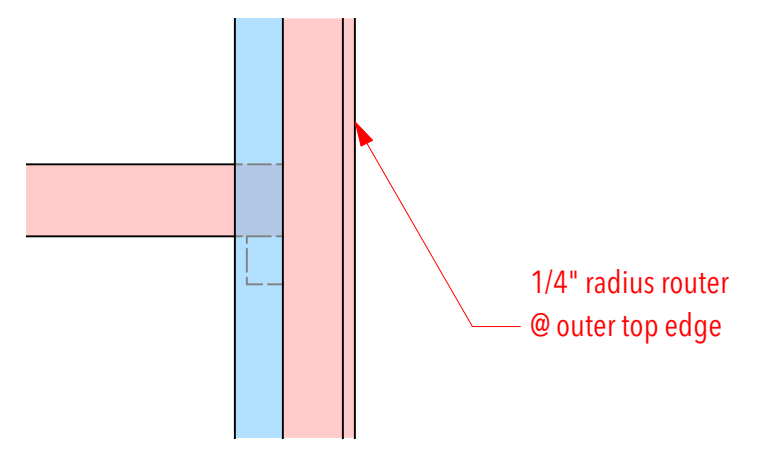
H-3 details Scale: 3" = 1'-0"
