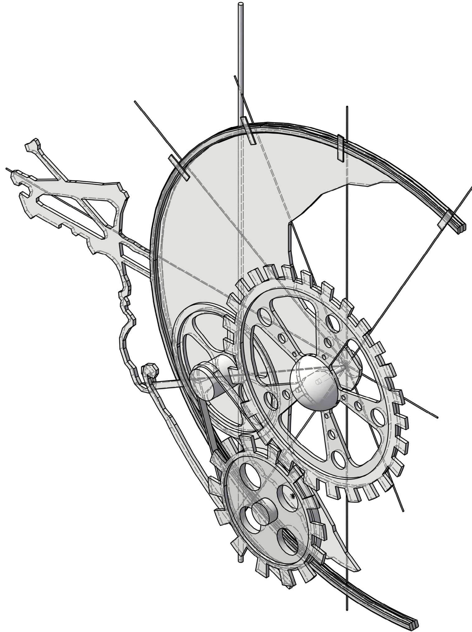
C-3 Clock SR: right isometric Scale: 1" = 1'-0"
