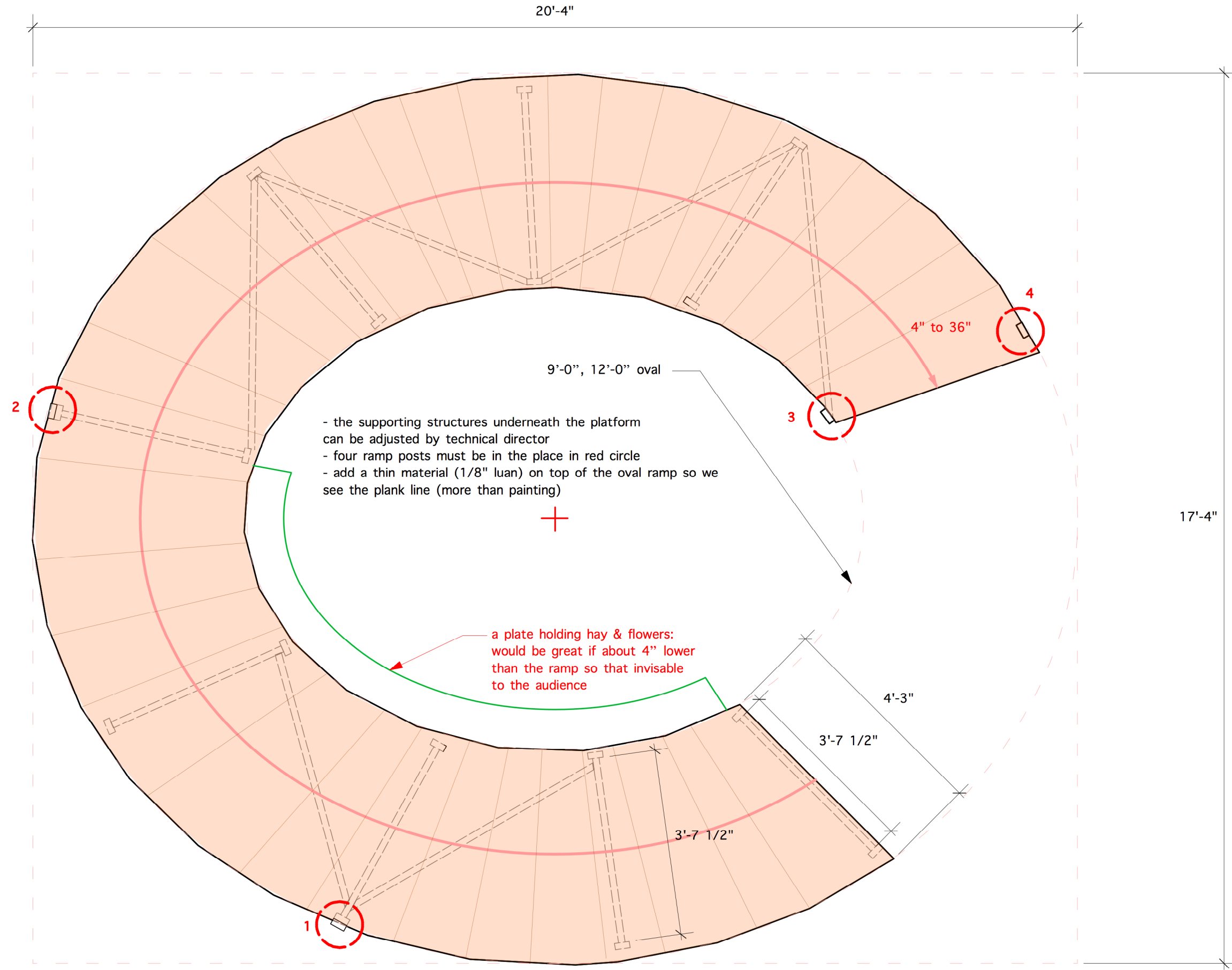
A-2 oval ramp: plan Scale: 1/2" = 1'-0"
