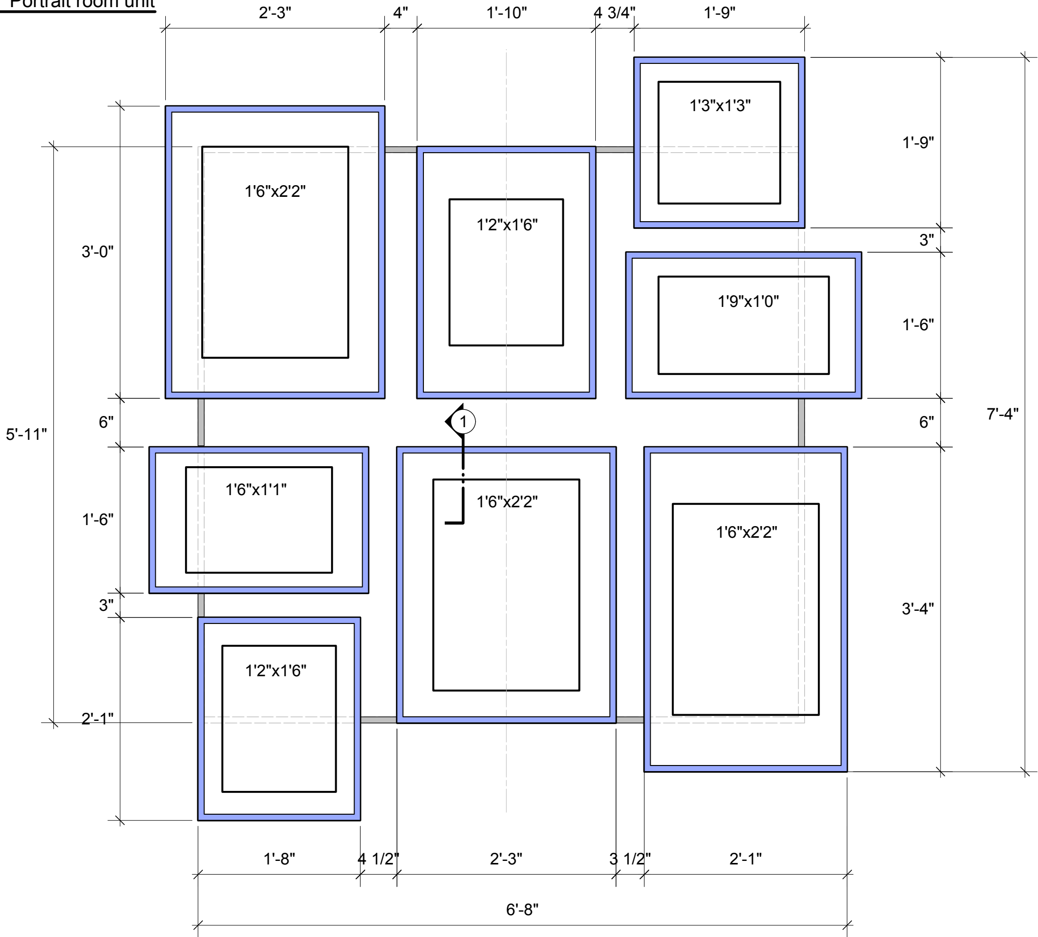
1 Portrait room unit Section scale: 1:1 (life scale)
