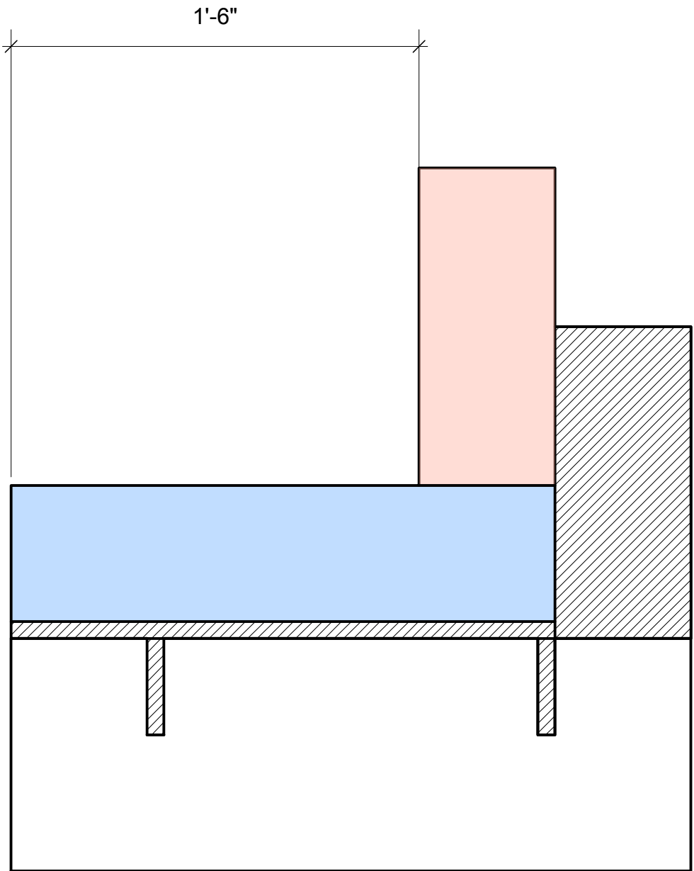
1 Section 1 Scale: 2" = 1'-0"
