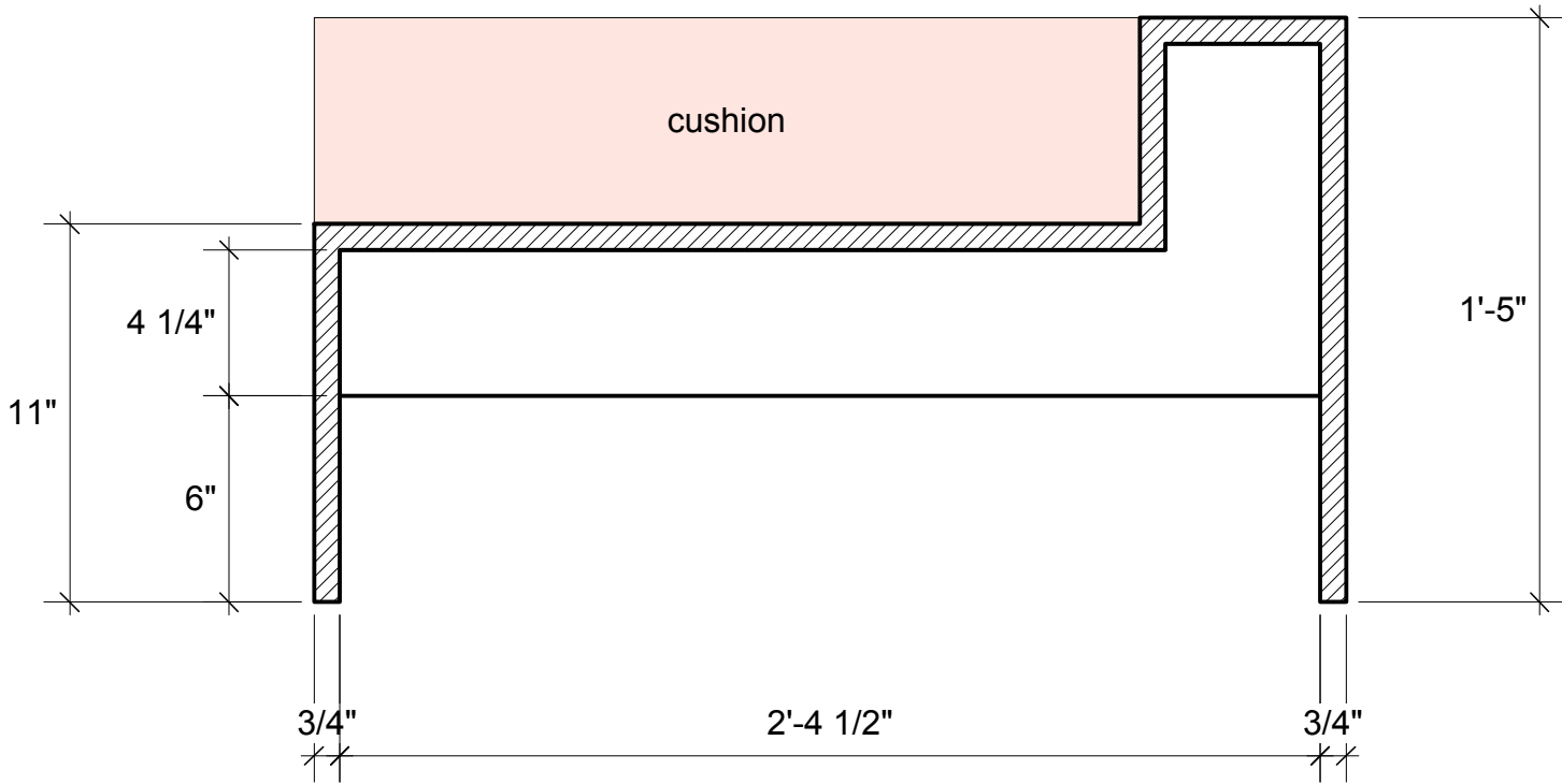
1 Section 1 Scale: 2" = 1'-0"
